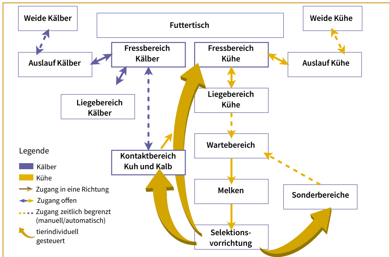
Funktionsschema für Verfahren der kuhgebundenen Kälberaufzucht mit Kurzzeitkontakt
