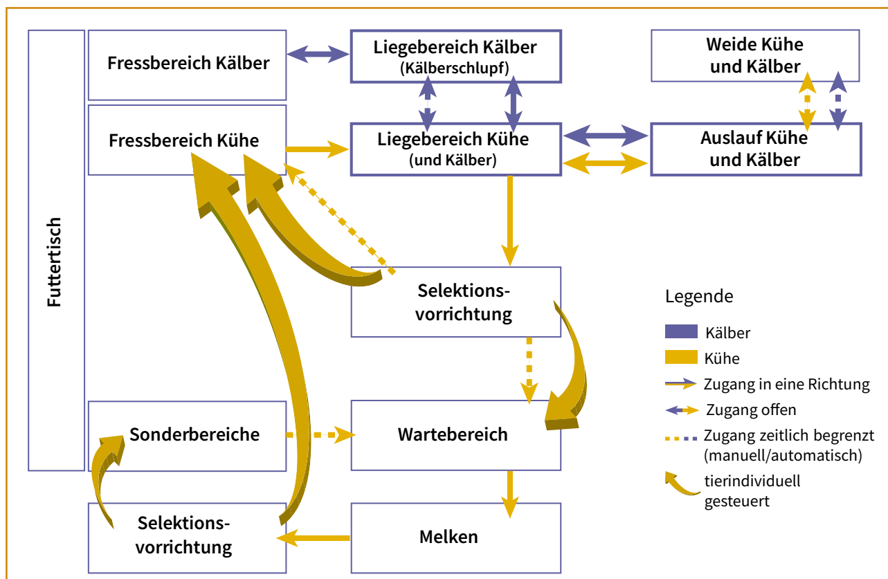
Funktionsschema für Verfahren mit Halb-/Ganztagskontakt, Kälberschlupf und selektivem Zugang zum Fress- bzw. Melkbereich
